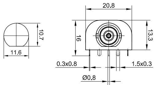
Bohrplan Panel drillings Perçages de panneau
